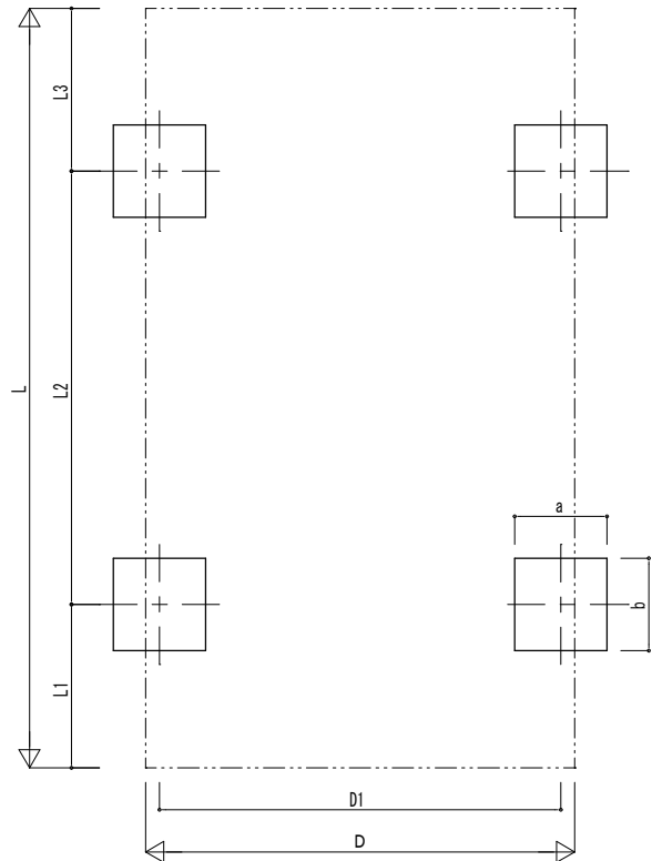
■基礎配置図
