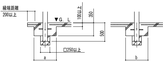
D ■基礎断面図
