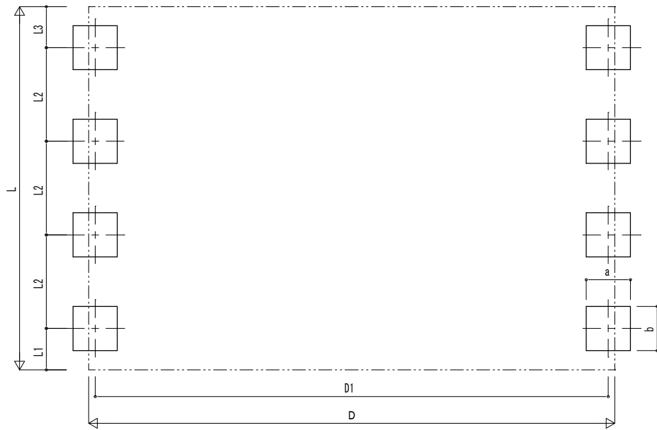
■基礎配置図
