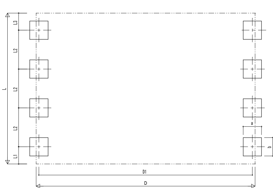
■基礎配置図
