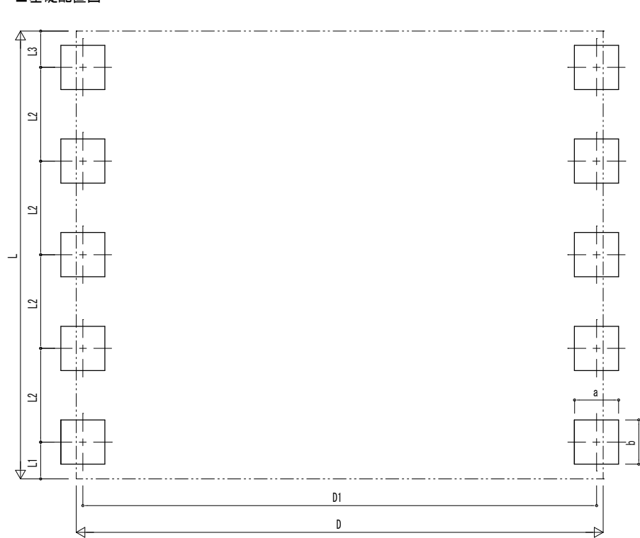
■基礎配置図
