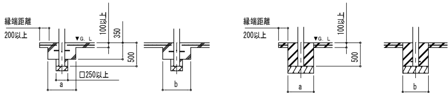
■基礎断面図
