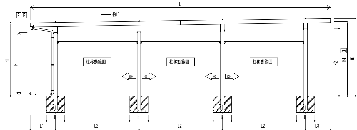
■ 基礎断面図
