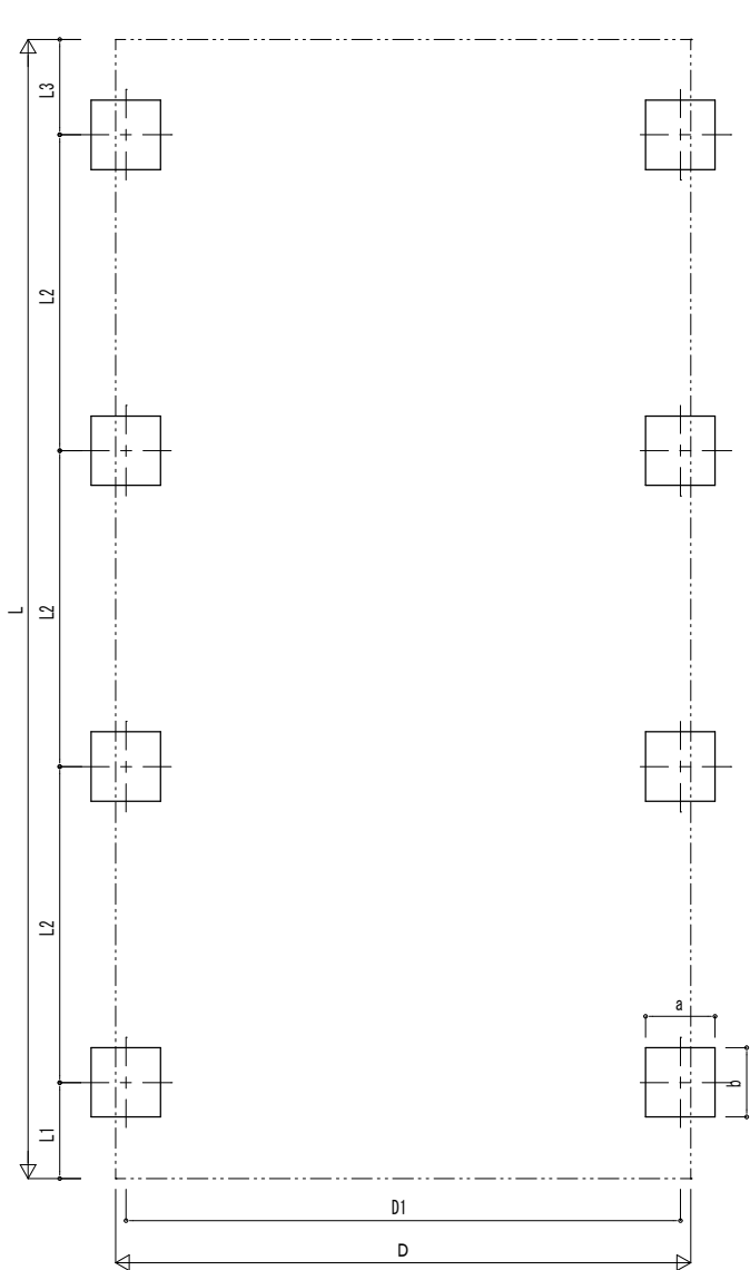
■ 基礎配置図
