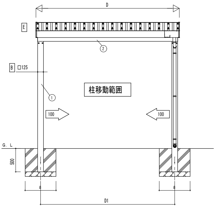
独立基礎の場合
