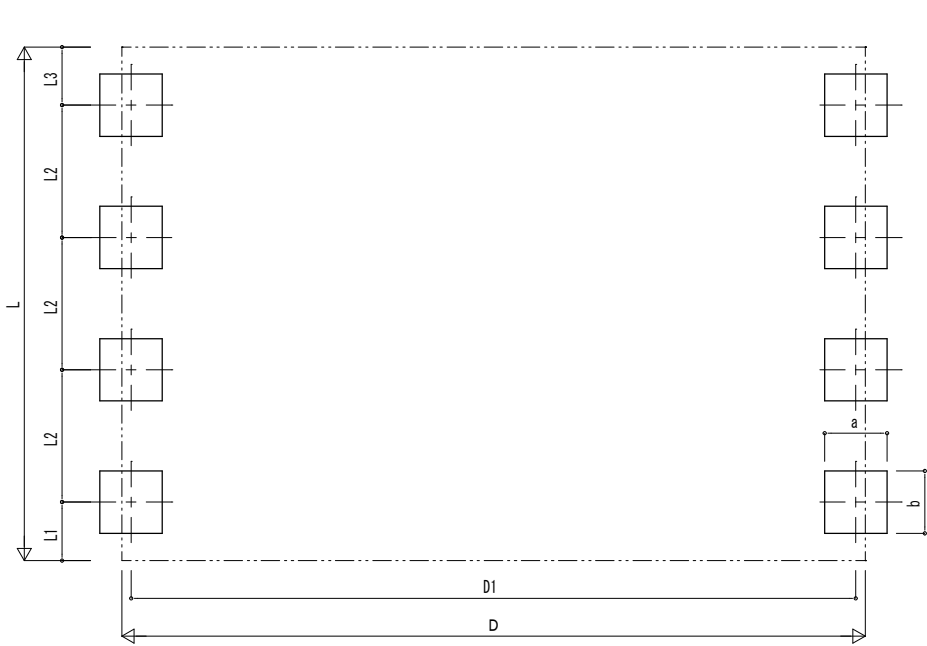
■ 基礎配置図
