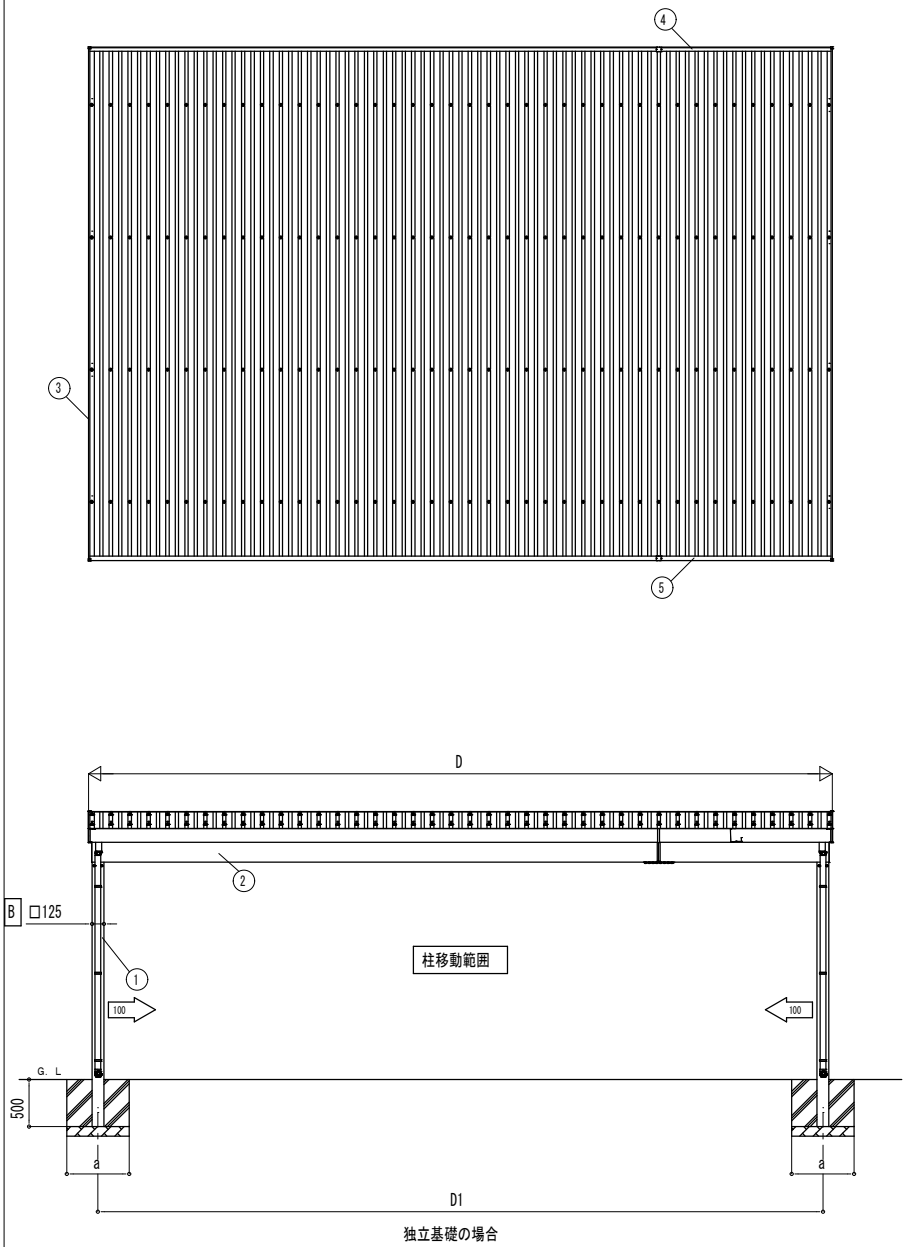
■ 姿図
