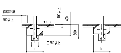
■ 基礎断面図
