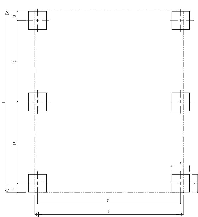
■ 基礎配置図
