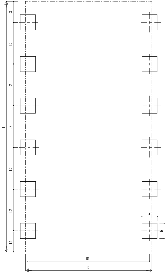
■ 基礎配置図
