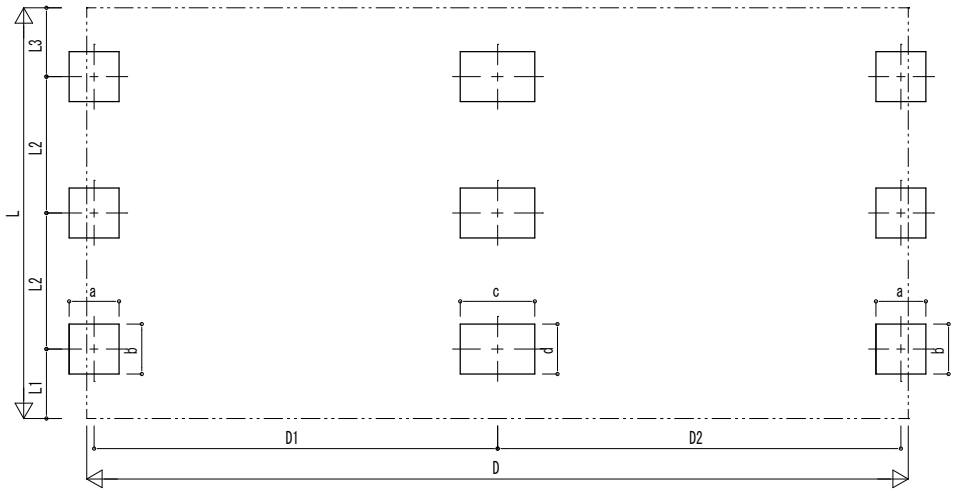
■基礎配置図
