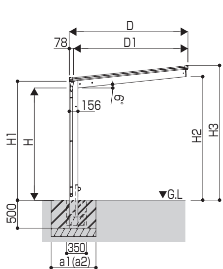
図は、独立基礎の場合を示します。
