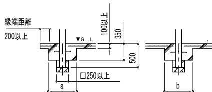
■ 基礎断面図
