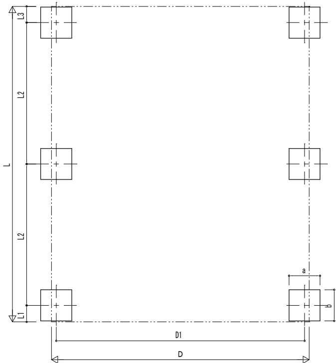
■ 基礎配置図
