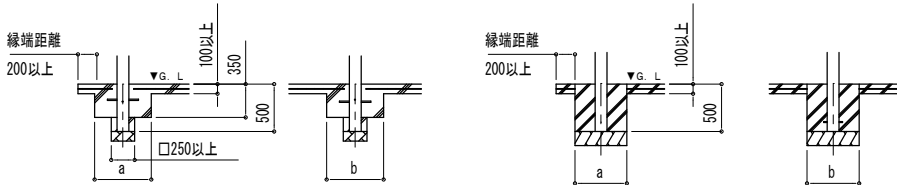
■ 基礎断面図
