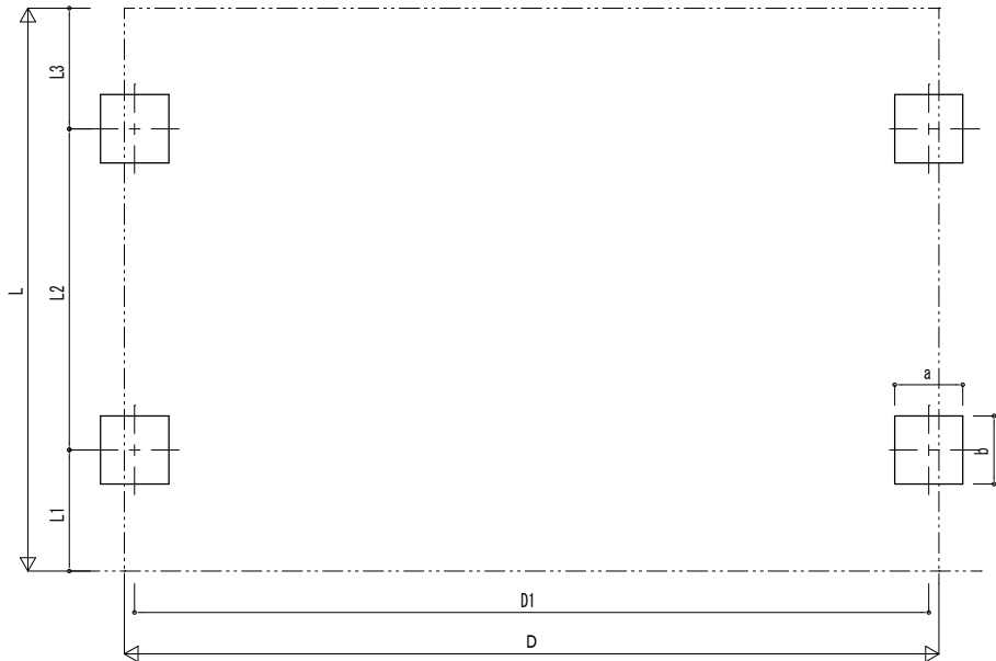
■ 基礎配置図
