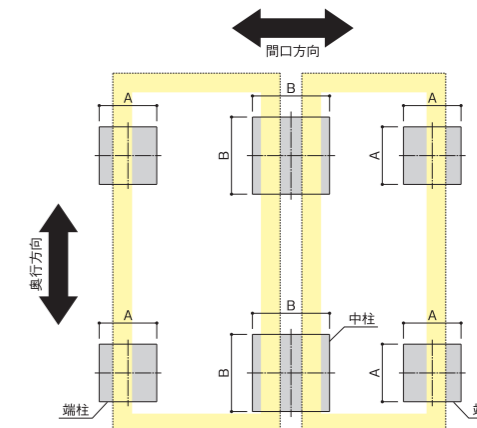
■横(2)連棟セット/基礎配置図
