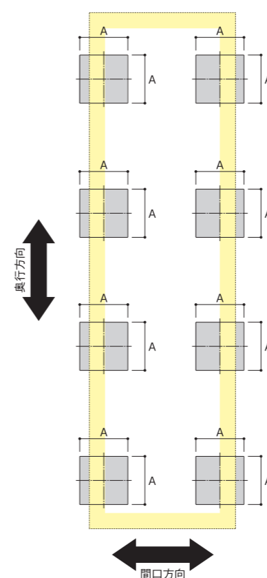
■たて(2)連棟セット/基礎配置図
