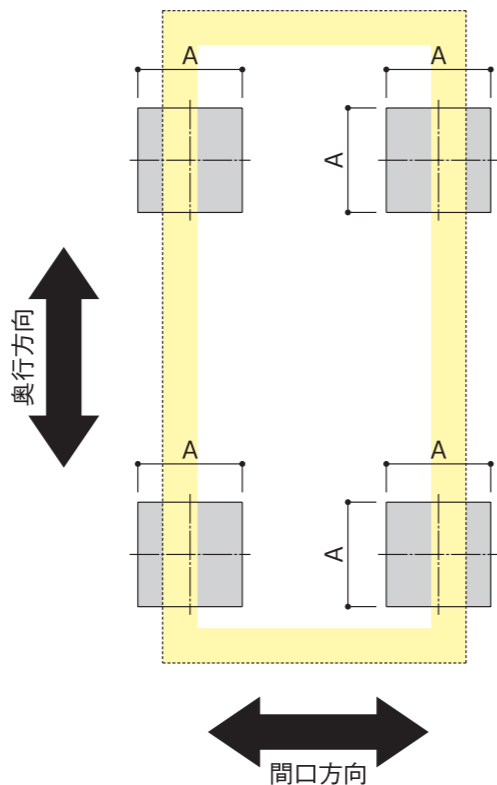
■基本セット・基礎配置図
